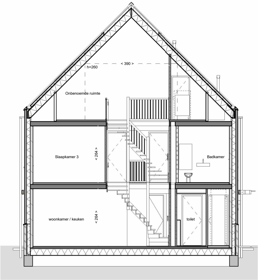
doorsnede
