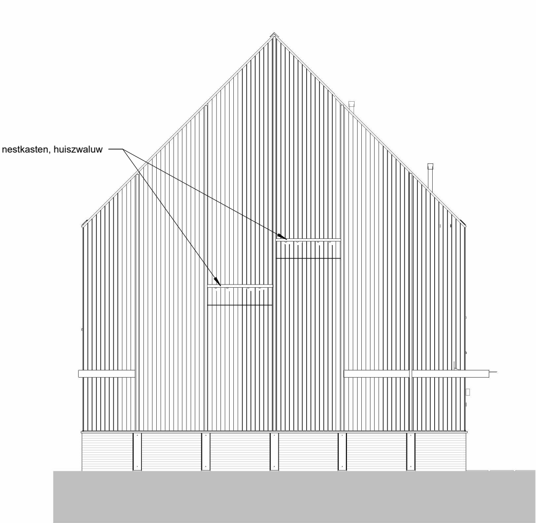
kopgevel
