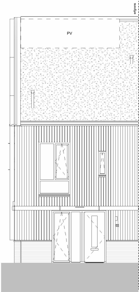
voorgevel
